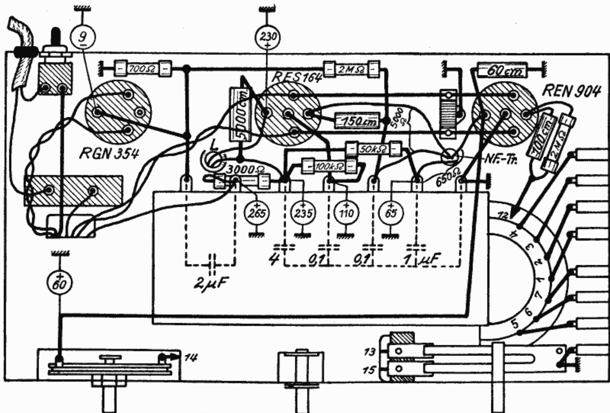
Verdrahtungsplan und Einzelteilanordnung des VE 301 W alt (Die eingekreisten Zahlen geben die Spannungen an).
