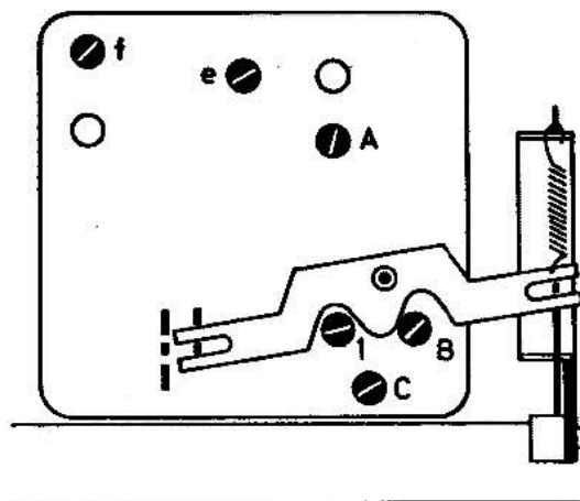
Mischteil von unten gesehen
